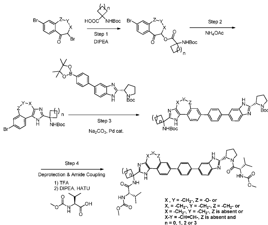
Scheme VI
