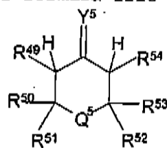
(IIIe)
