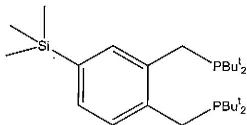
1,2-bis(di-tert-butyl(phosphinomethyl))-4-trimethylsilyl benzene
