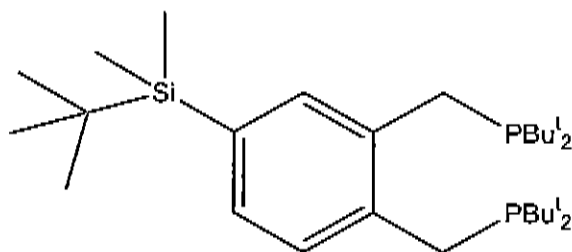
1,2-bis(di-tert-butyl(phosphinomethyl))-4-(tert-butyl dimethylsilyl) benzene
