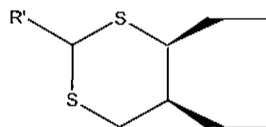
2 - substituted 1,3 dithiane
