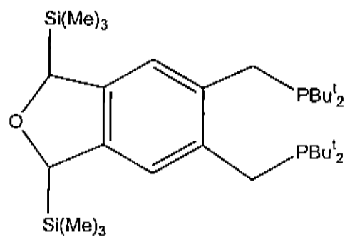
1,2-bis(di-tert-butylphosphinomethyl)-1'-tert-butyl ferrocene
