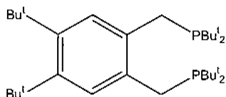
1,2-bis(di-tert-butyl(phosphinomethyl))-4,5-di-tert-butylbenzene
