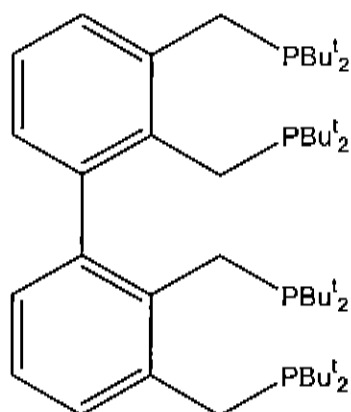
1,2-bis(di-tert-butyl(phosphinomethyl))-3-(2',3'-bis(di-tert-butyl(phosphinomethyl))phenyl)benzene
