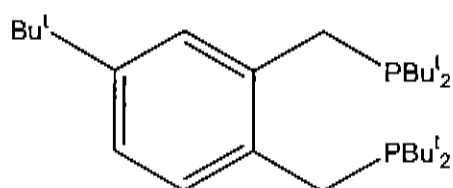
1,2-bis(di-tert-butyl(phosphinomethyl))-4-tert-butylbenzene
