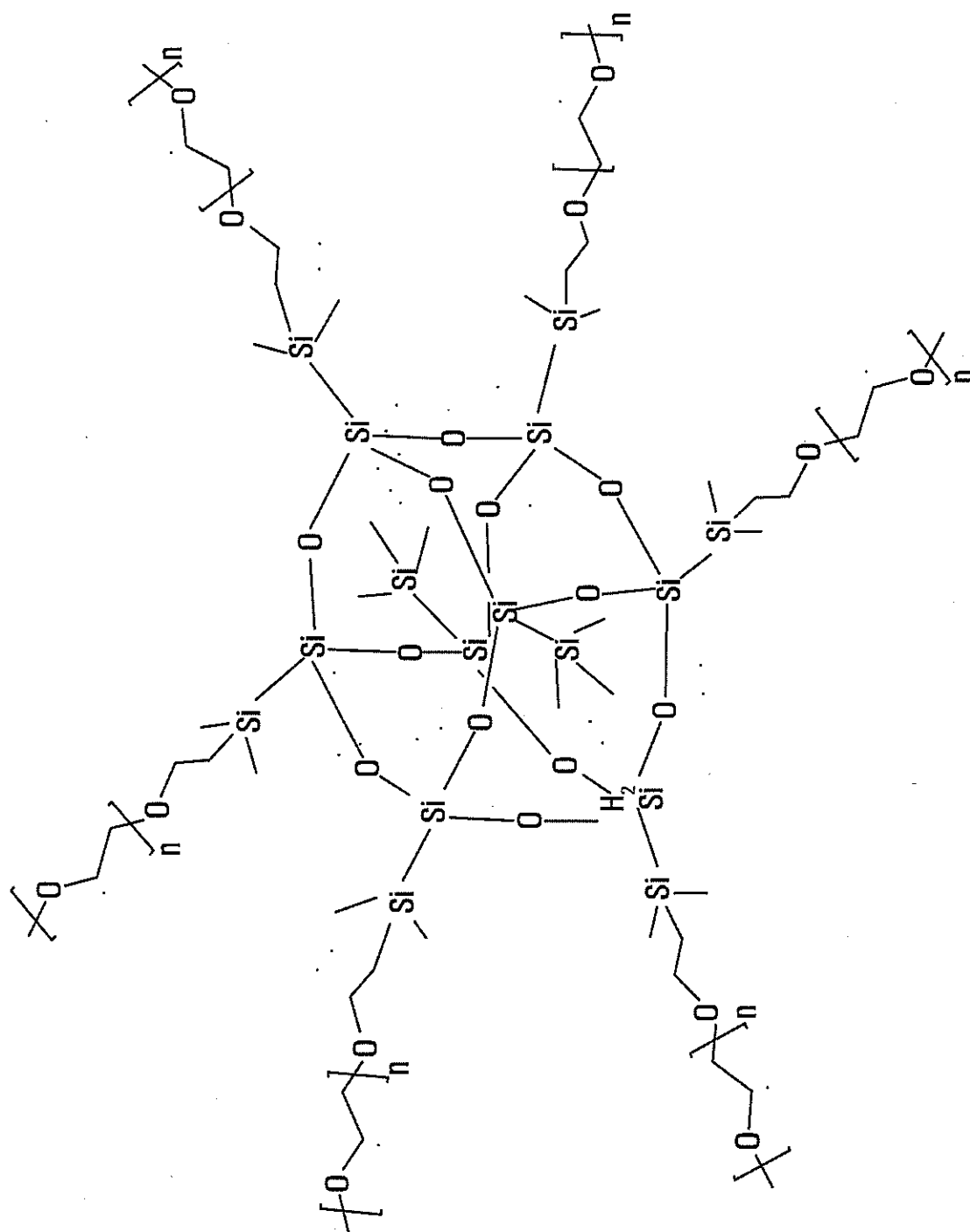
POSS-PEO
