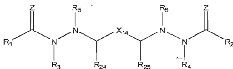
(XV)
