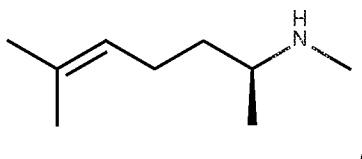
(S)-Isometheptene
