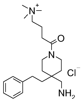
A.53 (Starting material: B.46)
