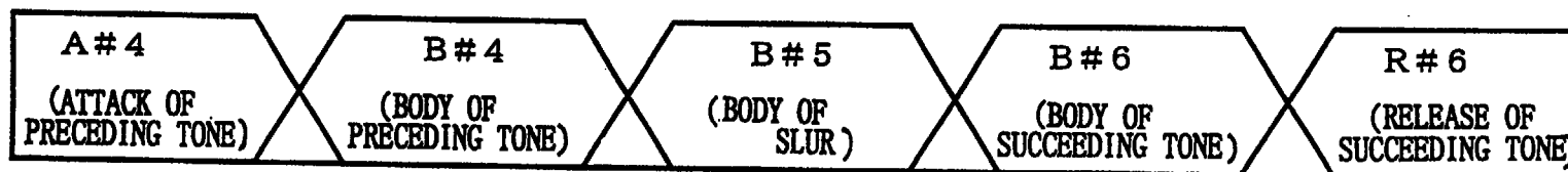
FIG. 9 C
