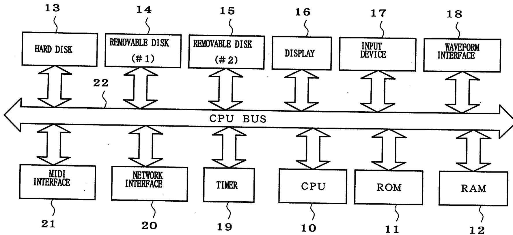
FIG. 22
