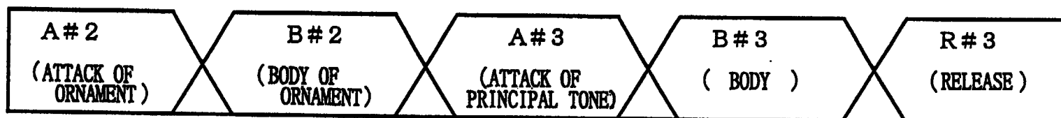
FIG. 9 B
