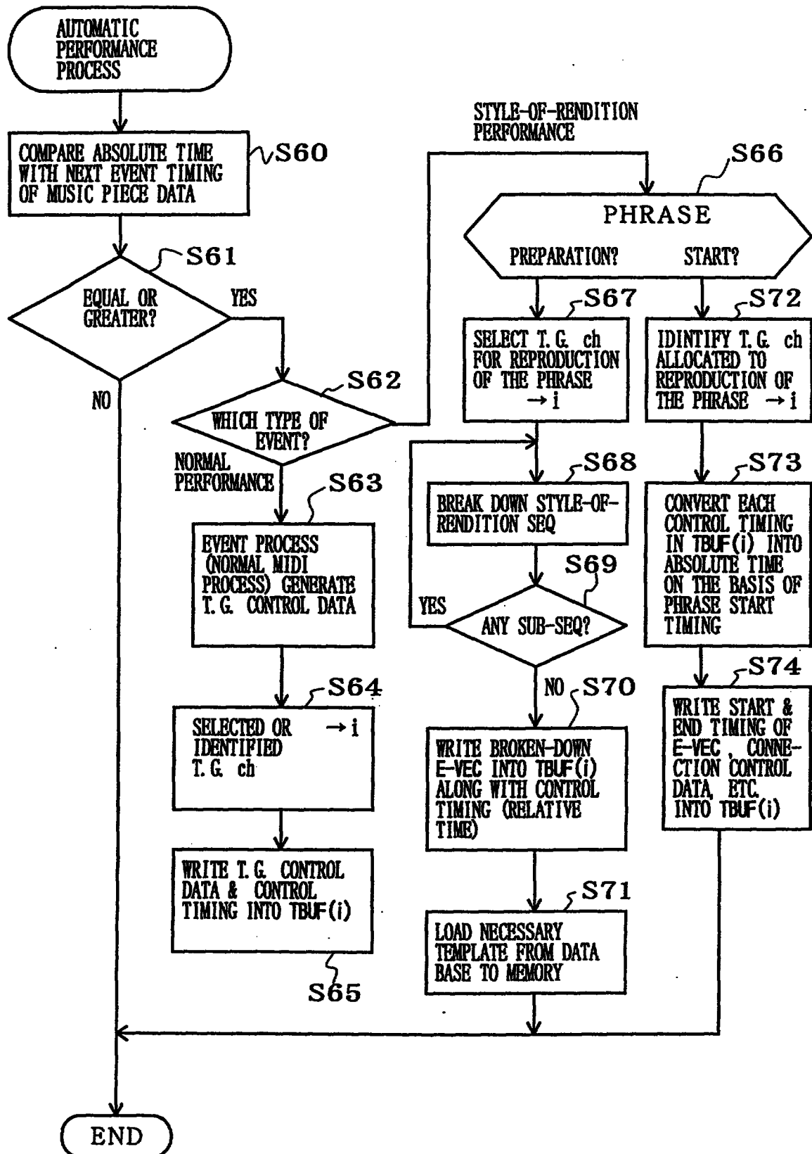
FIG. 27
