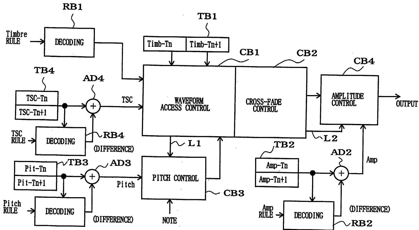
FIG. 21
