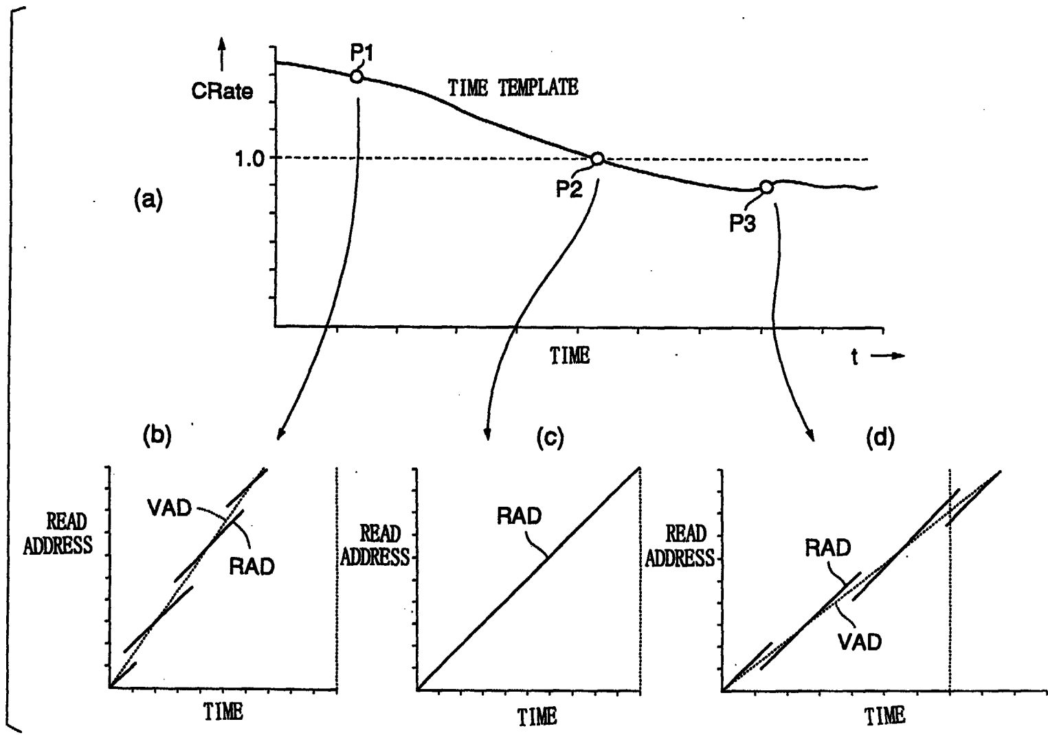
FIG. 31
