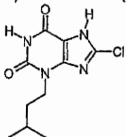
b) 8-chloro-3-(3-methylbutyl)-3,7-dihydro-1H-purine-2,6-dione
