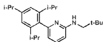
Ligand 3
