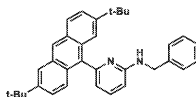
Ligand 6
