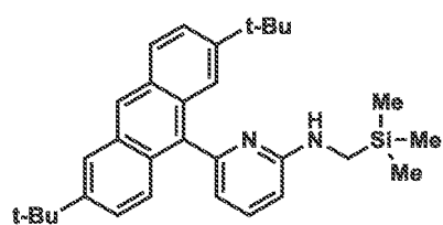
Ligand 7
