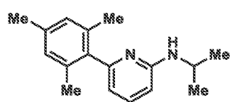
Ligand 5
