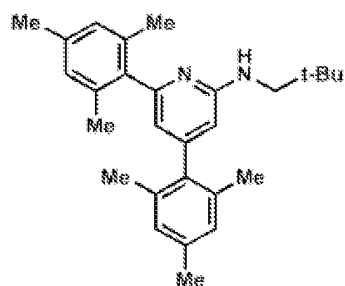
Ligand 2
