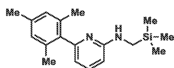
Ligand 4
