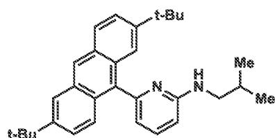
Ligand 8
