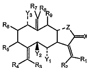
Formula Ic
