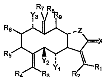
Formula Ic
