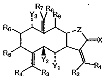
Formula Ic
