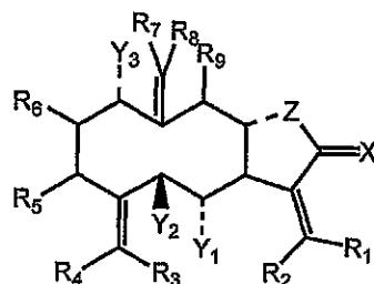
Formula Ic
