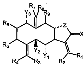
Formula Ic
