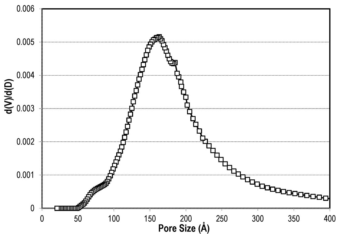
FIG. 6 Pore Diameter vs. d(V)/d(D)
