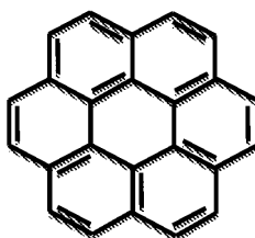
Coronene
