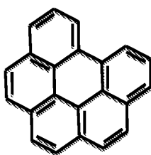
Benzoperylene
