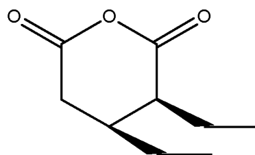
glutaric anhydride
