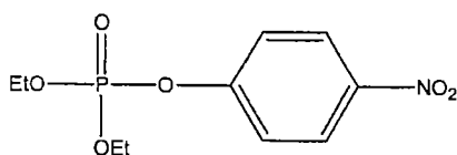
Paraoxon
