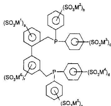
(IIa)
