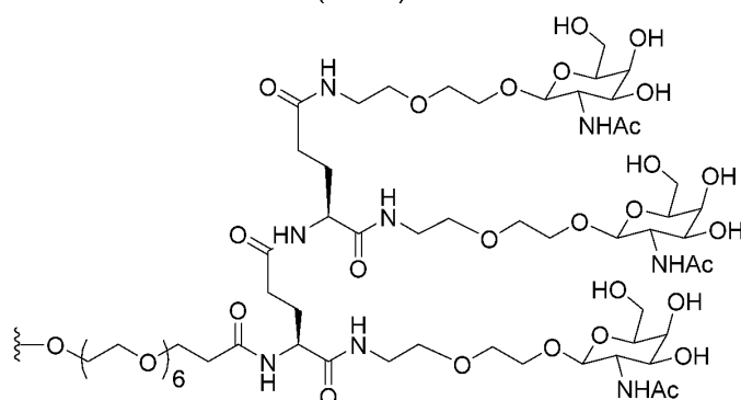
GalNAc(A5GN)
