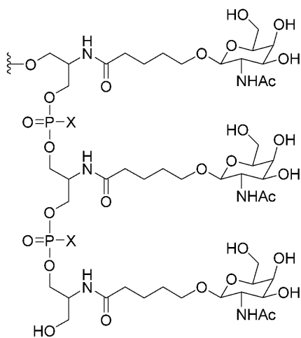
GalNAc(Ser1)
