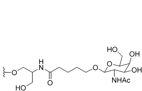
GalNAc(Ser1)
