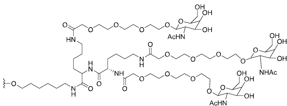
GalNAc(A5GN)
