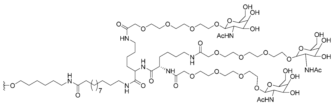
GalNAc(A3GN)
