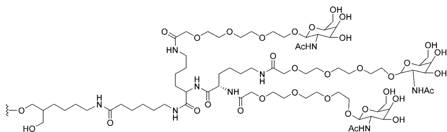
GalNAc(A1GN)
