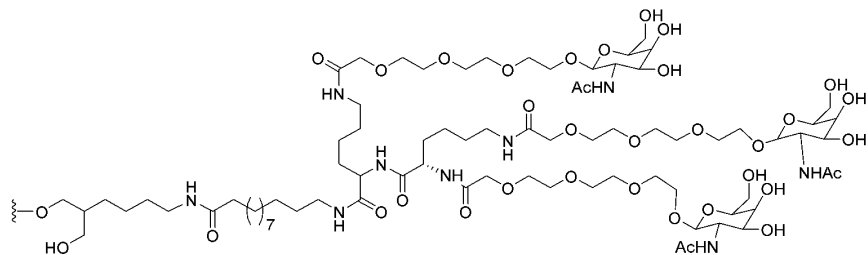
GalNAc(A2GN)
