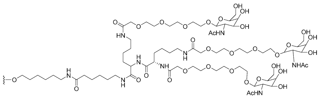
GalNAc(Ser3)
