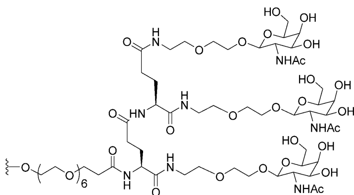
GalNAc(A5GN)
