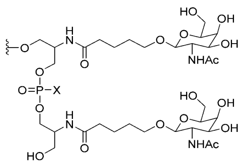
GalNAc(Ser2)
