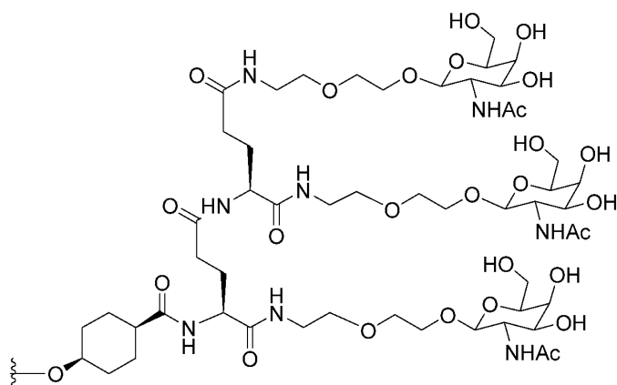
GalNAc(NAG37)
