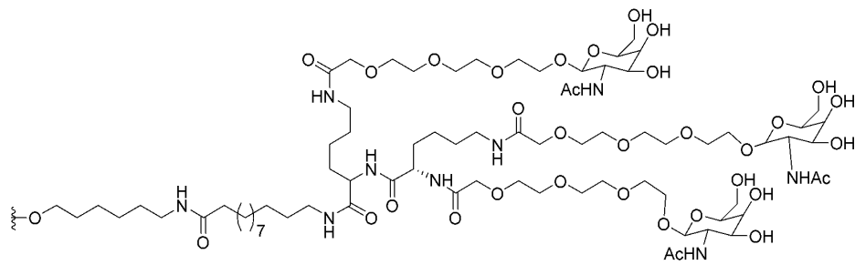
GalNAc(A3GN)
