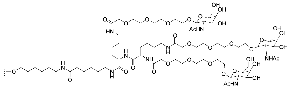
GalNAc(A2GN)
