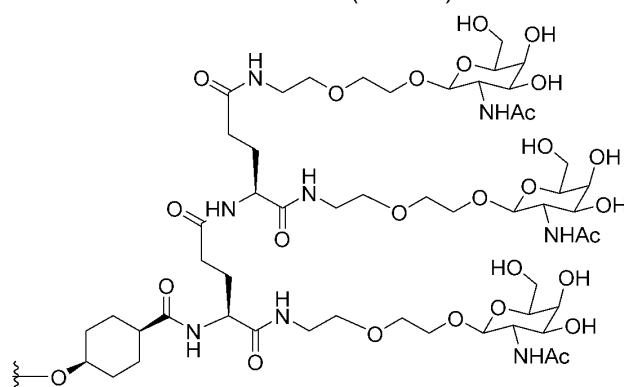
GalNAc(NAG37)
