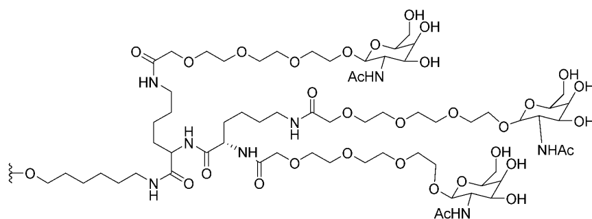
GalNAc(A5GN)
