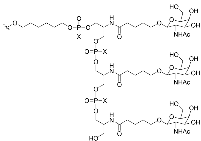
GalNAc(Ser3)
