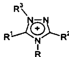
(IVg'')
