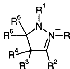
(IVj)
