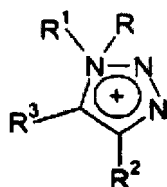
(IVr)
