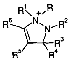
(IVk)
