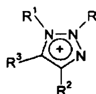
(IVr')
