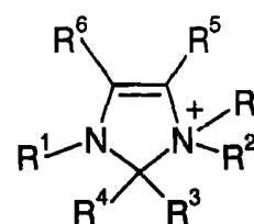
(IVl)
