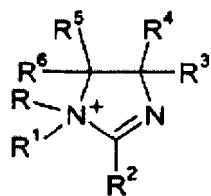
(IVm')
