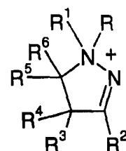
(IVj')
