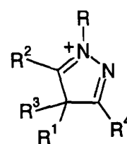
(IVh)
