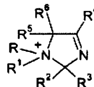
(IVn')
