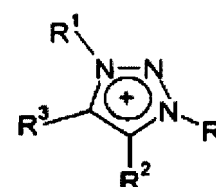
(IVr'')
