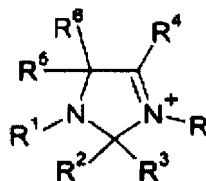
(IVn)
