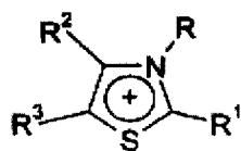
(IVo)
