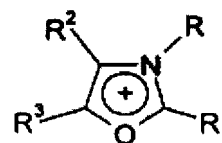
(IVp)
