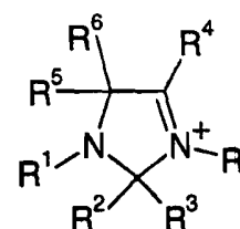
(IVn)
