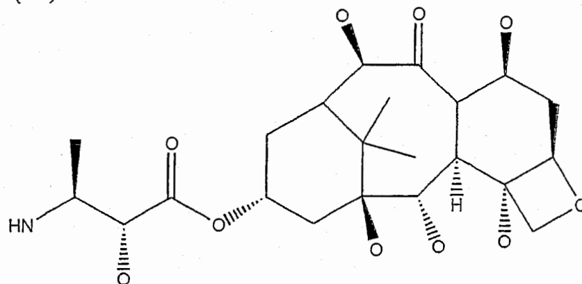
(VII).
