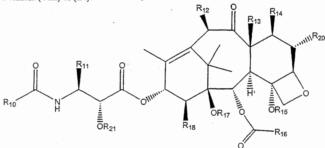
(VIII).
