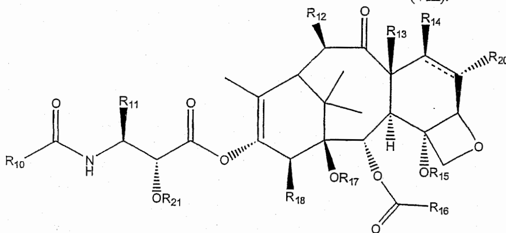
(VIII).
