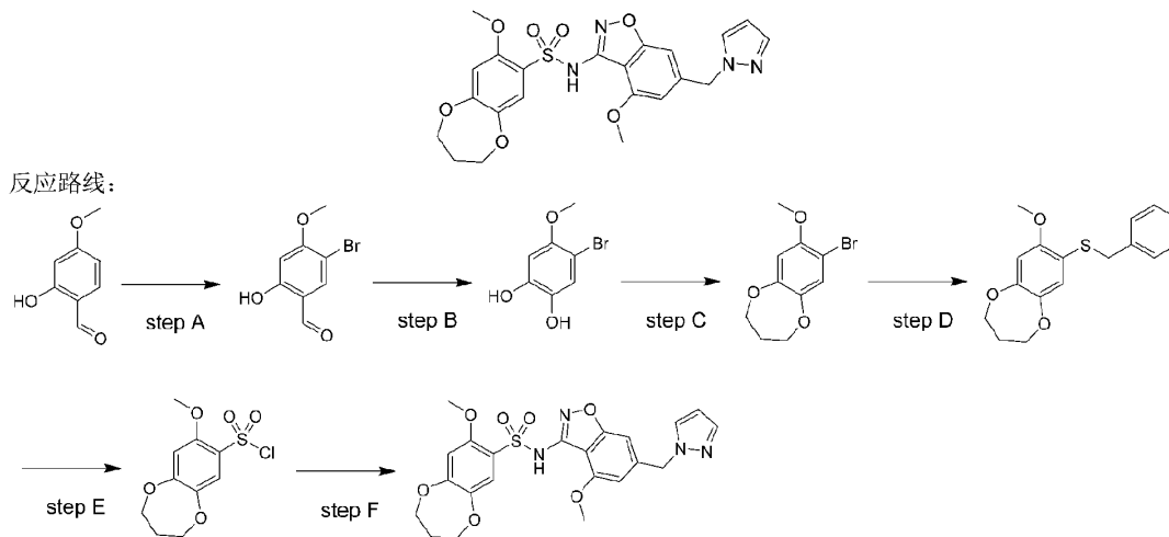
化合物7
