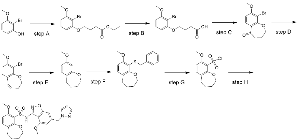
化合物16
