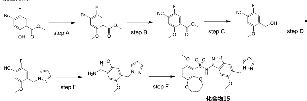
化合物15
