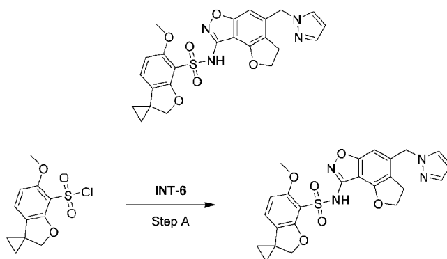
化合物36
