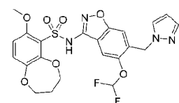
化合物 13
