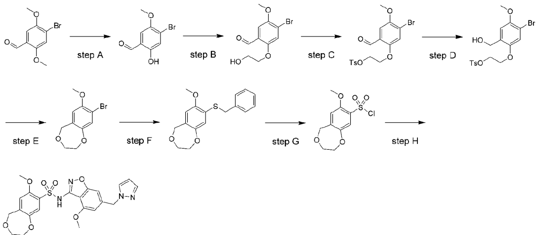
化合物8
