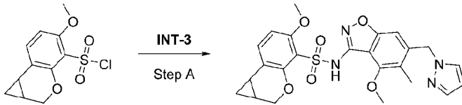
化合物24
