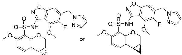
化合物30-P1
