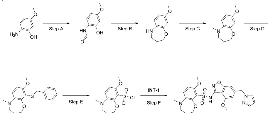
化合物41
