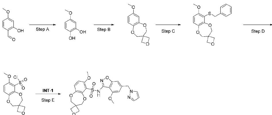
化合物32
