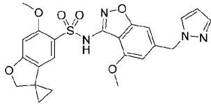
化合物4
