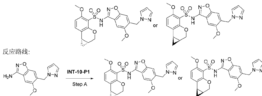
化合物33
