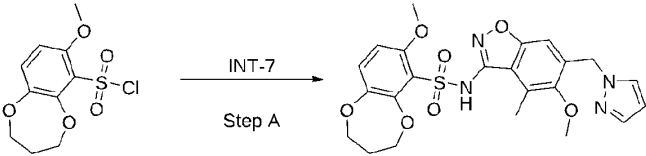
化合物38
