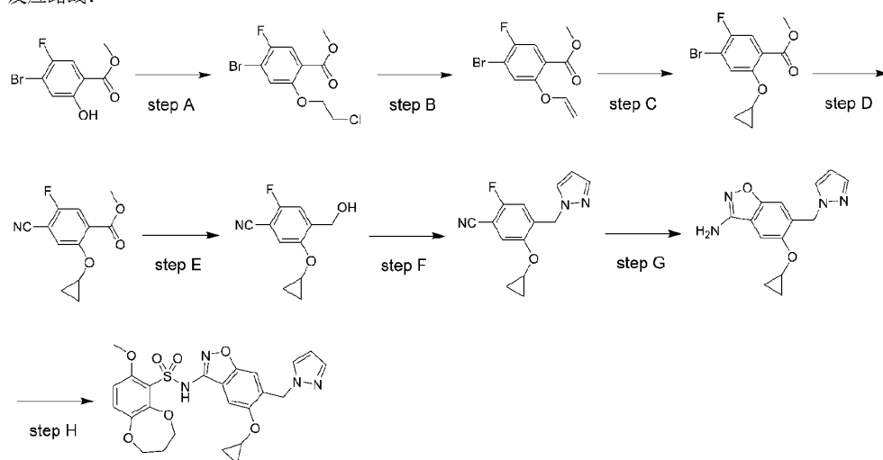
化合物19
