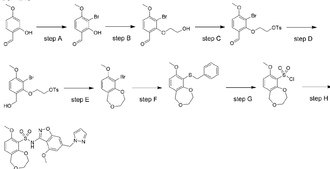
化合物 10
