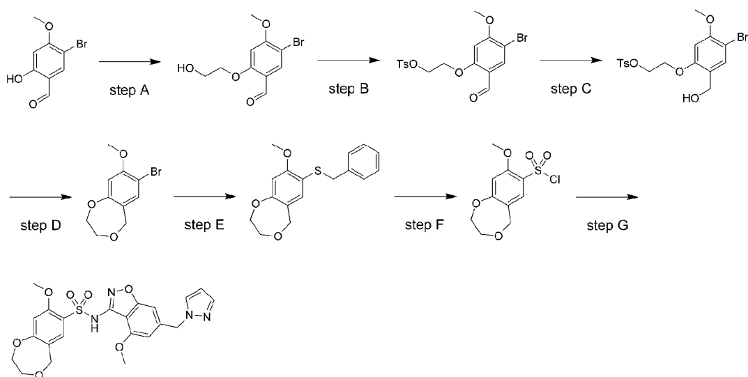
化合物9
