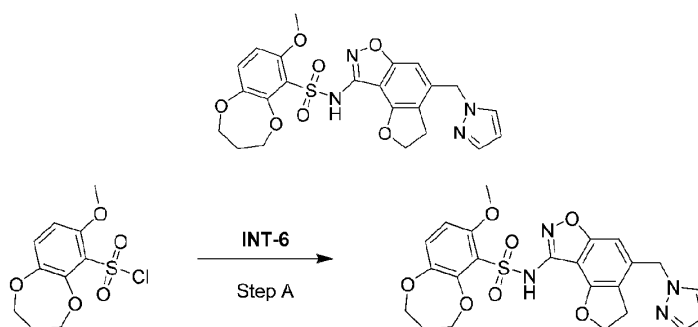
化合物35
