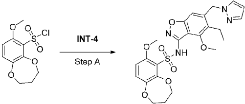
化合物26
