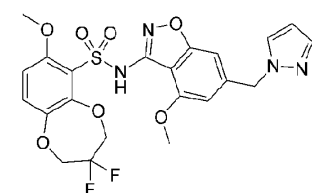
化合物11
