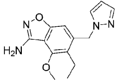
INT-4
