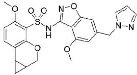
化合物5
