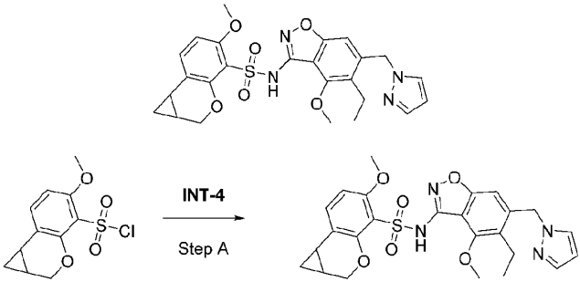
化合物27
