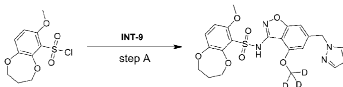
化合物46
