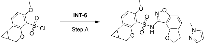
化合物37
