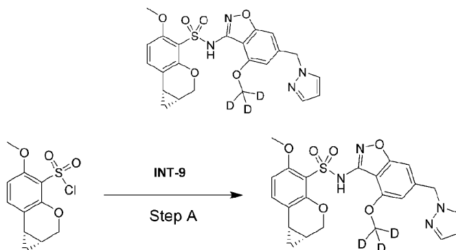
化合物45
