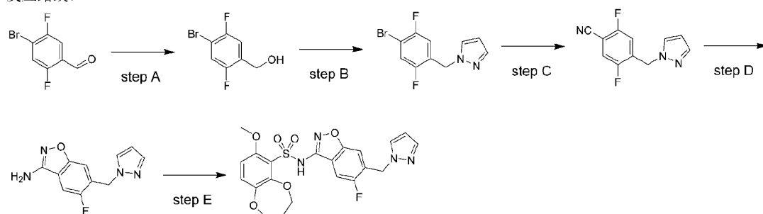
化合物 12
