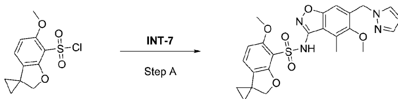
化合物39
