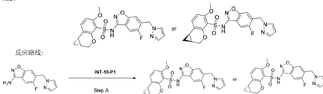
化合物34
