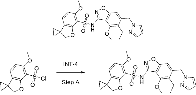
化合物28
