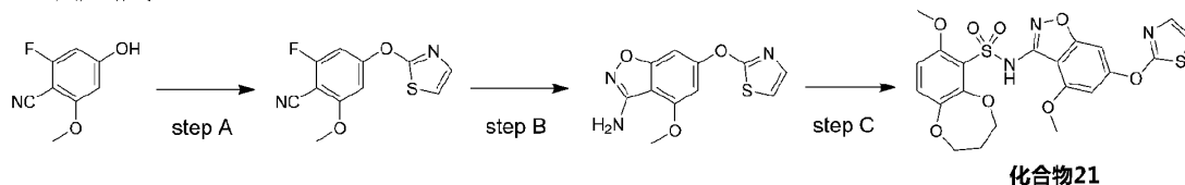
化合物21
