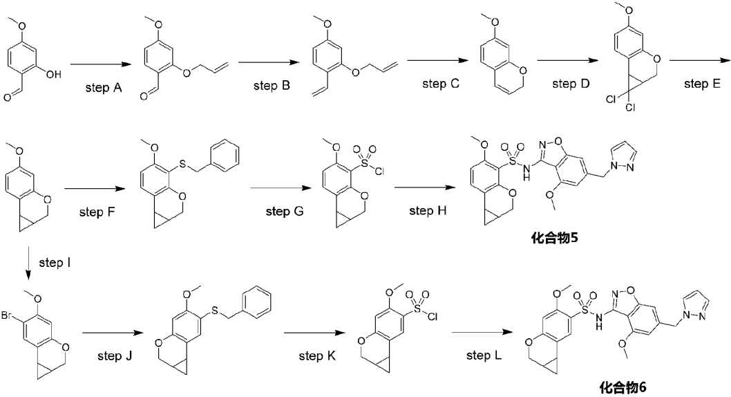
化合物6
