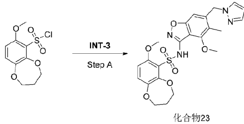
化合物23
