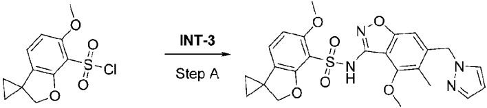
化合物25
