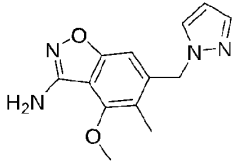
INT-3
