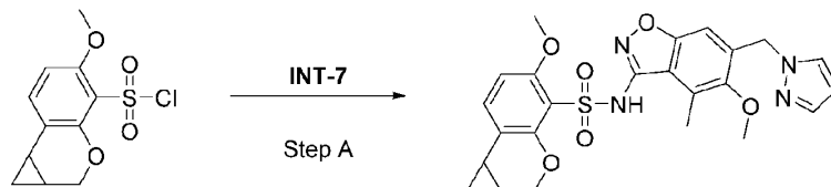
化合物40
