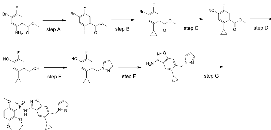
化合物14
