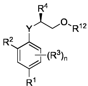
(M.XIV)
