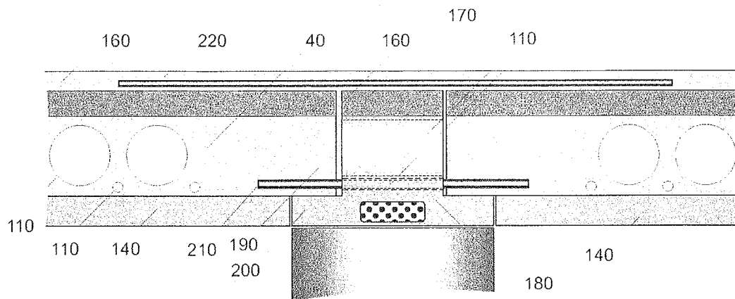
fig 11 cut a-a
