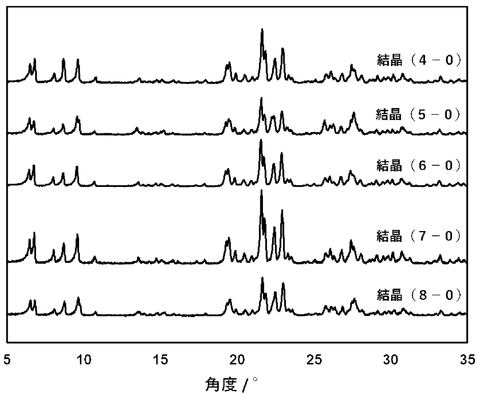
アルミノシリケートのXRDチャート
