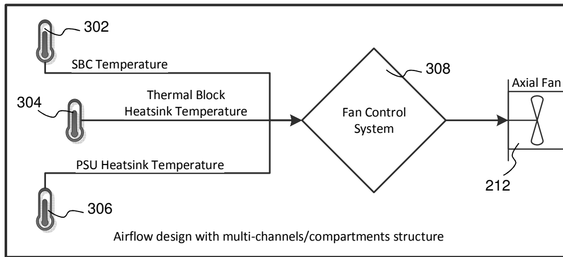
Fan Control Block Diagram
