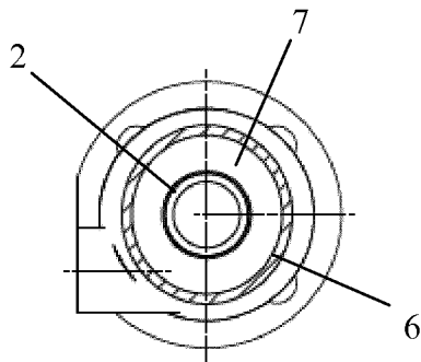
Fig. 6 Section D-D
