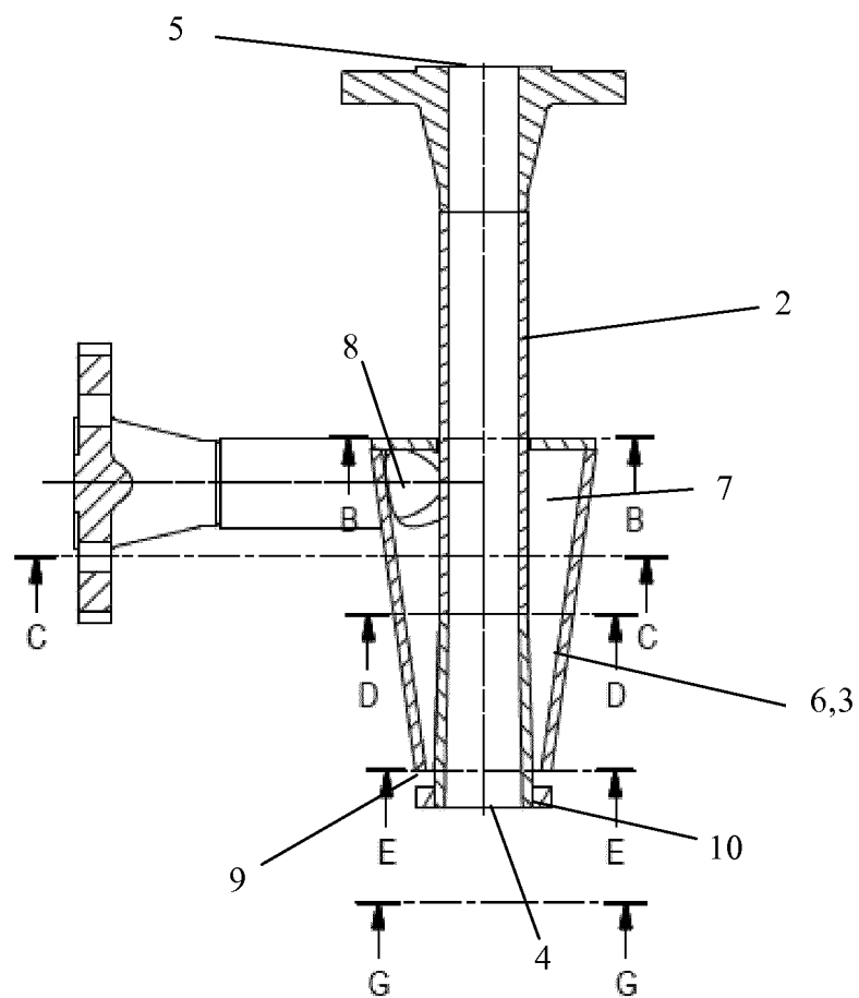
Fig. 3 Section A-A
