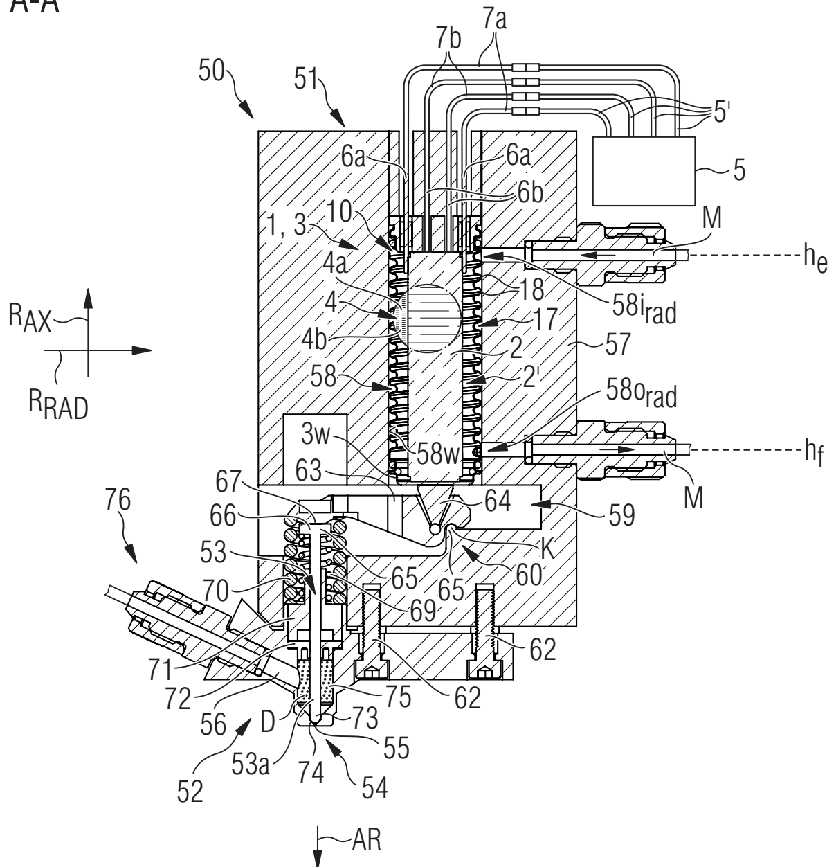
FIG 2 A-A
