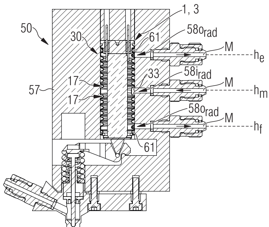
FIG 6 A"-A"
