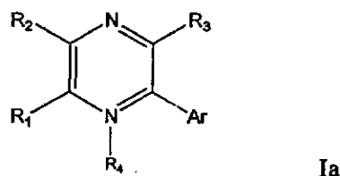
Ia
