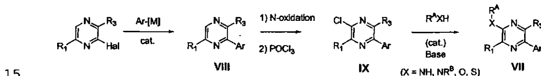
Scheme II (Method B)
