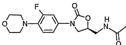
Linezolid
