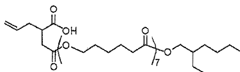
Macromonomer A5
