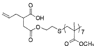
Macromonomer E5
