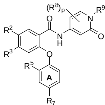
I-G
