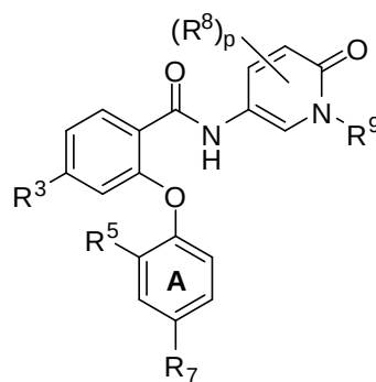
I'-F
