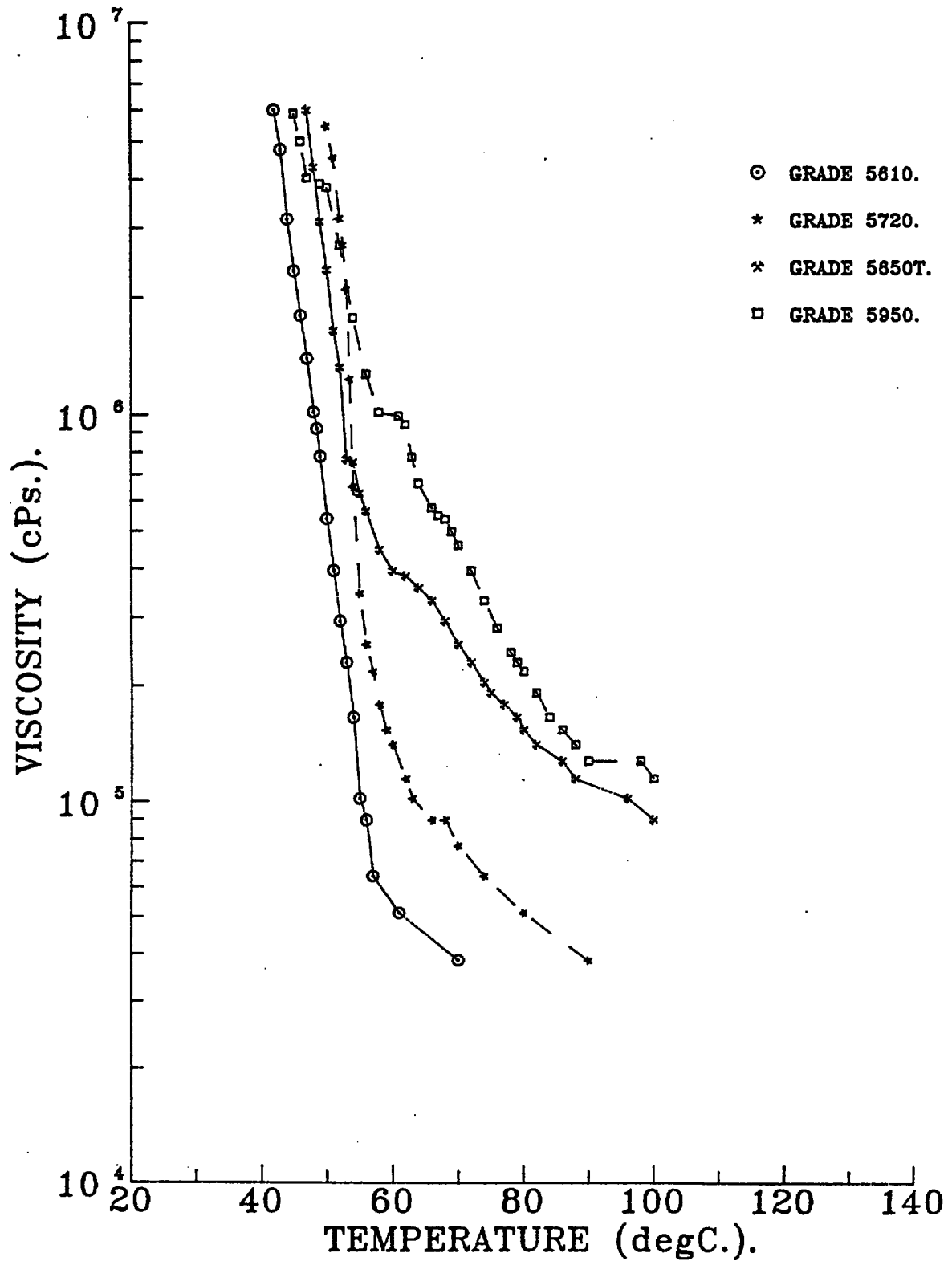
FIG 1:ELVAX-2 RESINS 40per.NVS. in ISOPAR L. (cooling curve).
