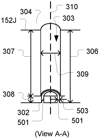
(View A-A) Fig. 5A-2
