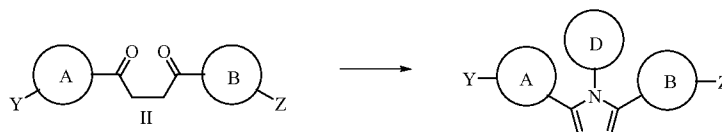
Scheme VI
