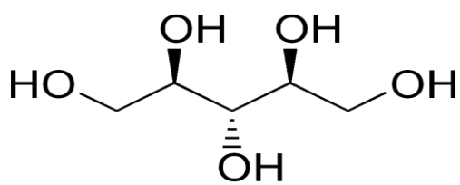
Ribitol,
