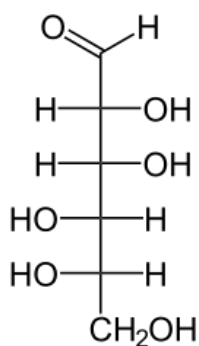
L-Mannose
