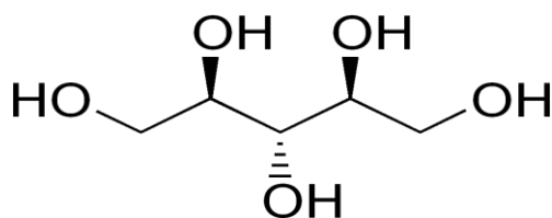
Ribitol,
