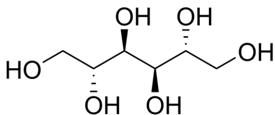
Mannitol,
