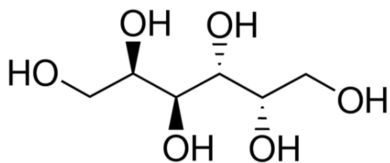
Dulcitol,
