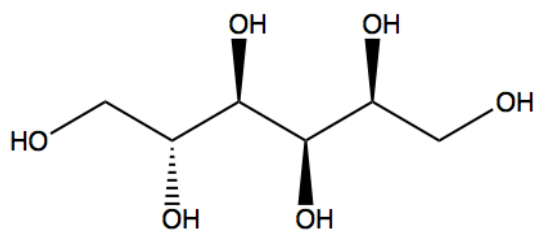
D-sorbitol,
