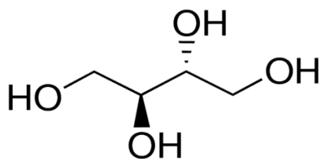
Meso-erythritol,
