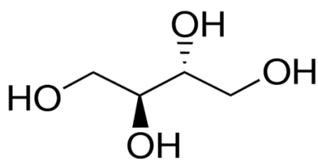
Meso-erythritol,
