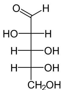
D-Arabinose
