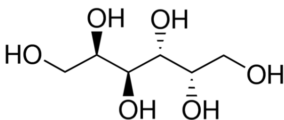
Dulcitol,
