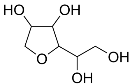
Sorbitan,
