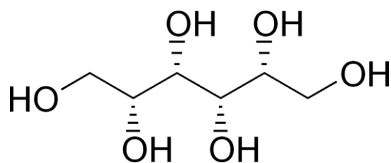
Iditol.
