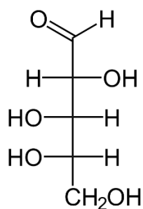
L-Arabinose
