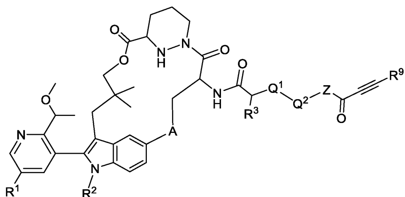
Formula II-6,
