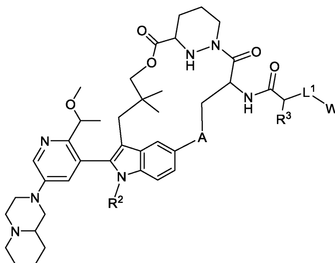
Formula II-4.
