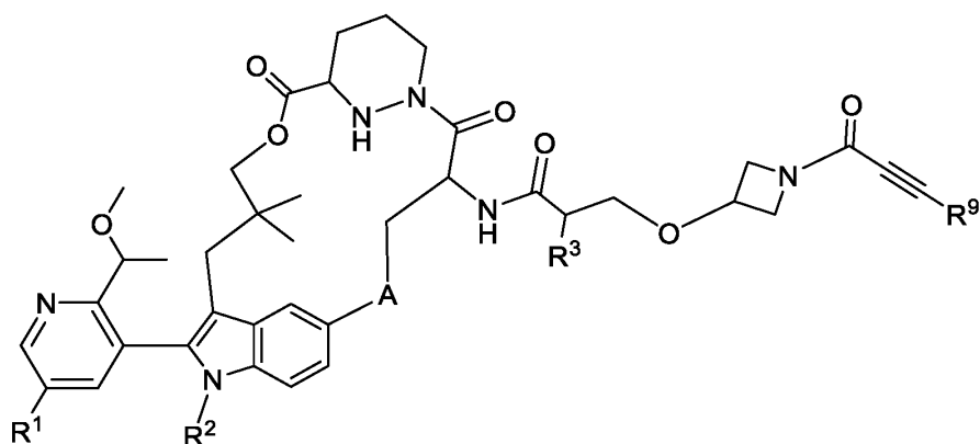
Formula II-6c.
