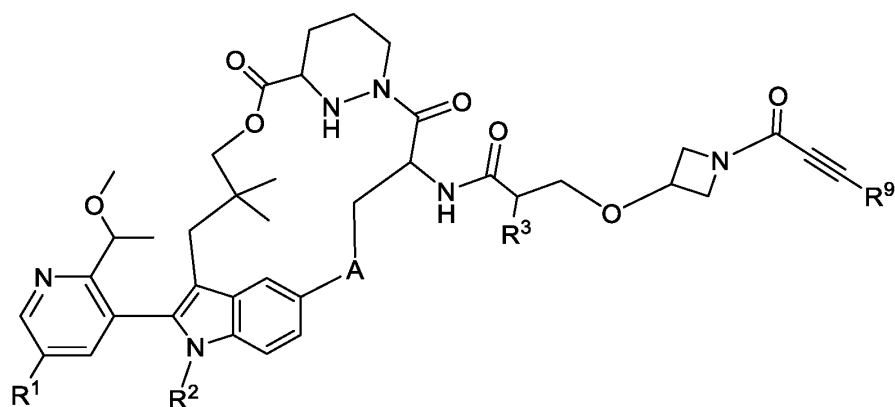
Formula II-6c.
