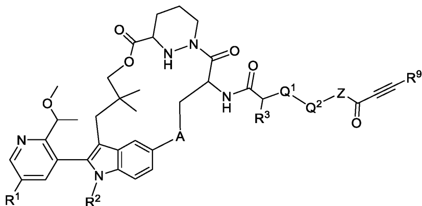
Formula II-6,
