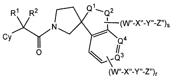
VII.
