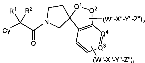
VII;
