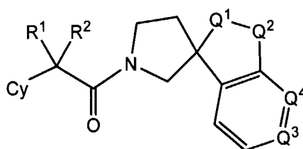
VIII;
