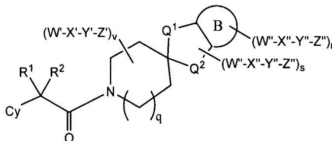
Va
