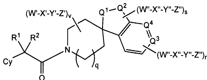
Vb
