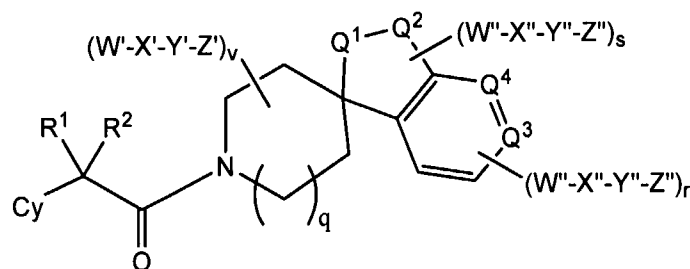
VI
