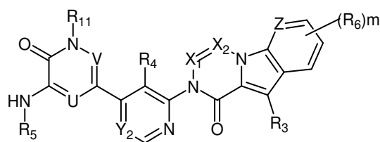
(IV)
