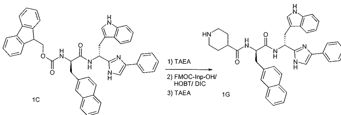
Scheme 1G
