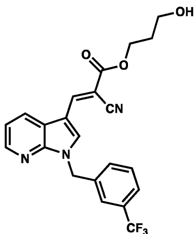
3-hydroxypropyl ( E )-2-cyano-3-(1-(3-(trifluoromethyl)benzyl)-1 H -pyrrolo[2,3- b ]pyridin-3-yl)acrylate
