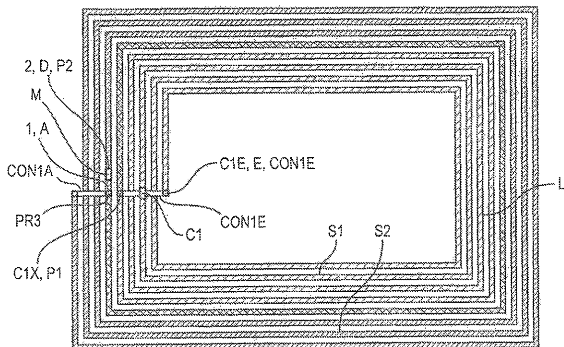
Antenne - 21AA
