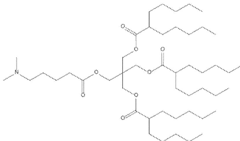
(化合物1)
