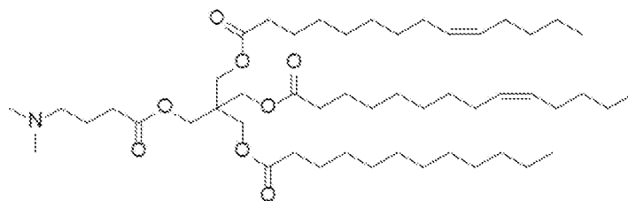
(化合物 21)
