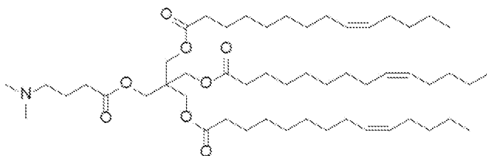
(化合物 11)
