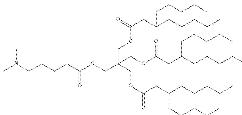
(化合物7)
