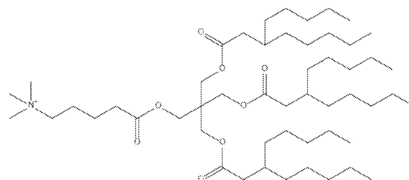
(化合物8)
