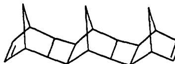
Norbornadiene Trimer
