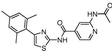
2-Acetamido-N-(4-mesitylthiazol-2-yl)isonicotinamide
