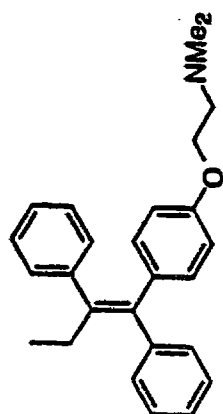
Iamoxifen
