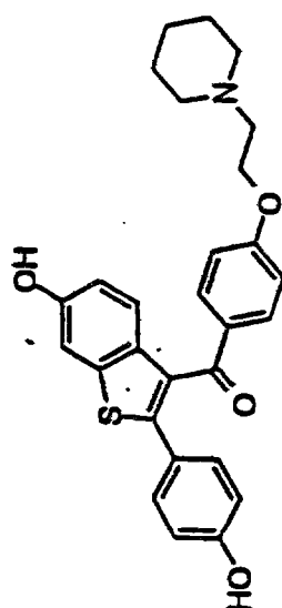
raloxifene
