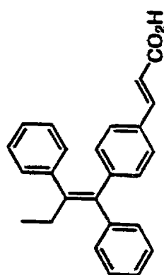
GW 5638
