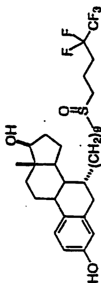
ICI 182780
