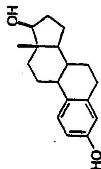
estradiol
