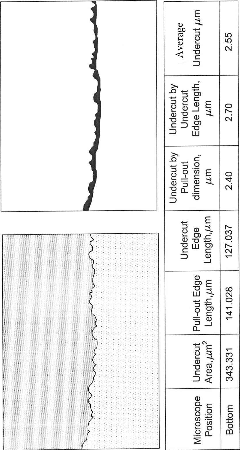
FIG. 12B
