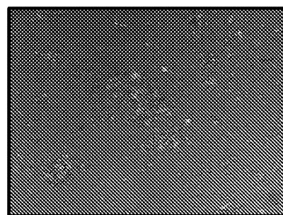
\text{H}_3\text{PO}_4 salt, Lot 6044-160-3
