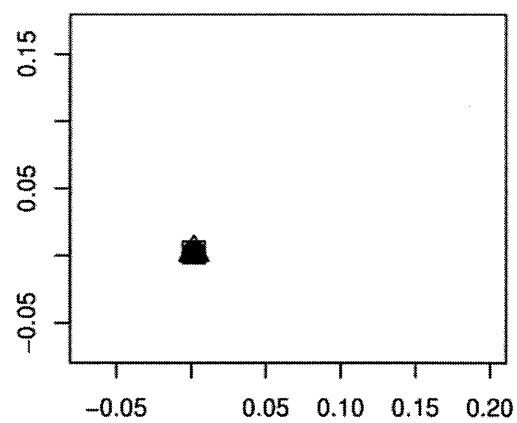
Abundant uniques only
