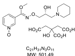
Methoxylated ORZY-04 (RRT 0.74)
