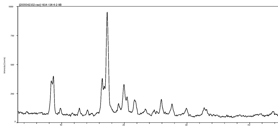
FIG. 11 XRPD Form Va
