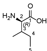
D-isoleucine (dl)
