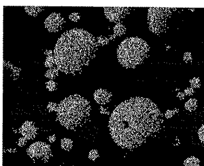
Mo La1
