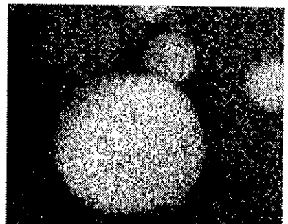
Mo La1
