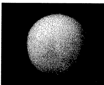
O Ka1
