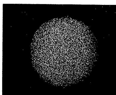
Al Ka1
