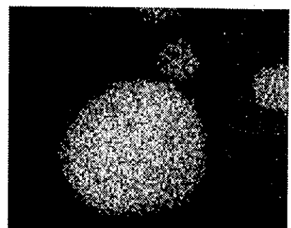
Al Ka1
