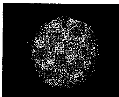
Mo La1
