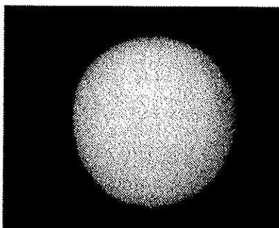
Si Ka1
