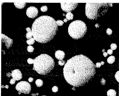
Si Ka1
