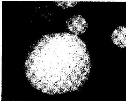
Si Ka1
