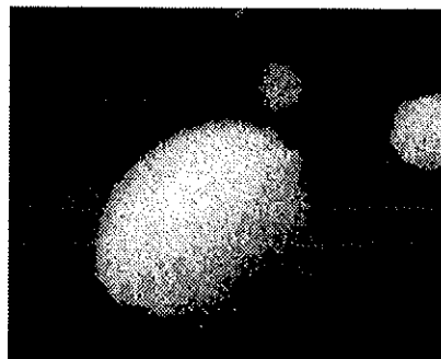
O Ka1
