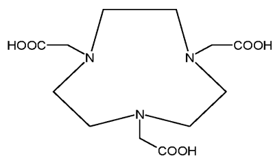
H 3 NOTA (comp.)
