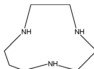
Triazacyclodecane (TACD)
